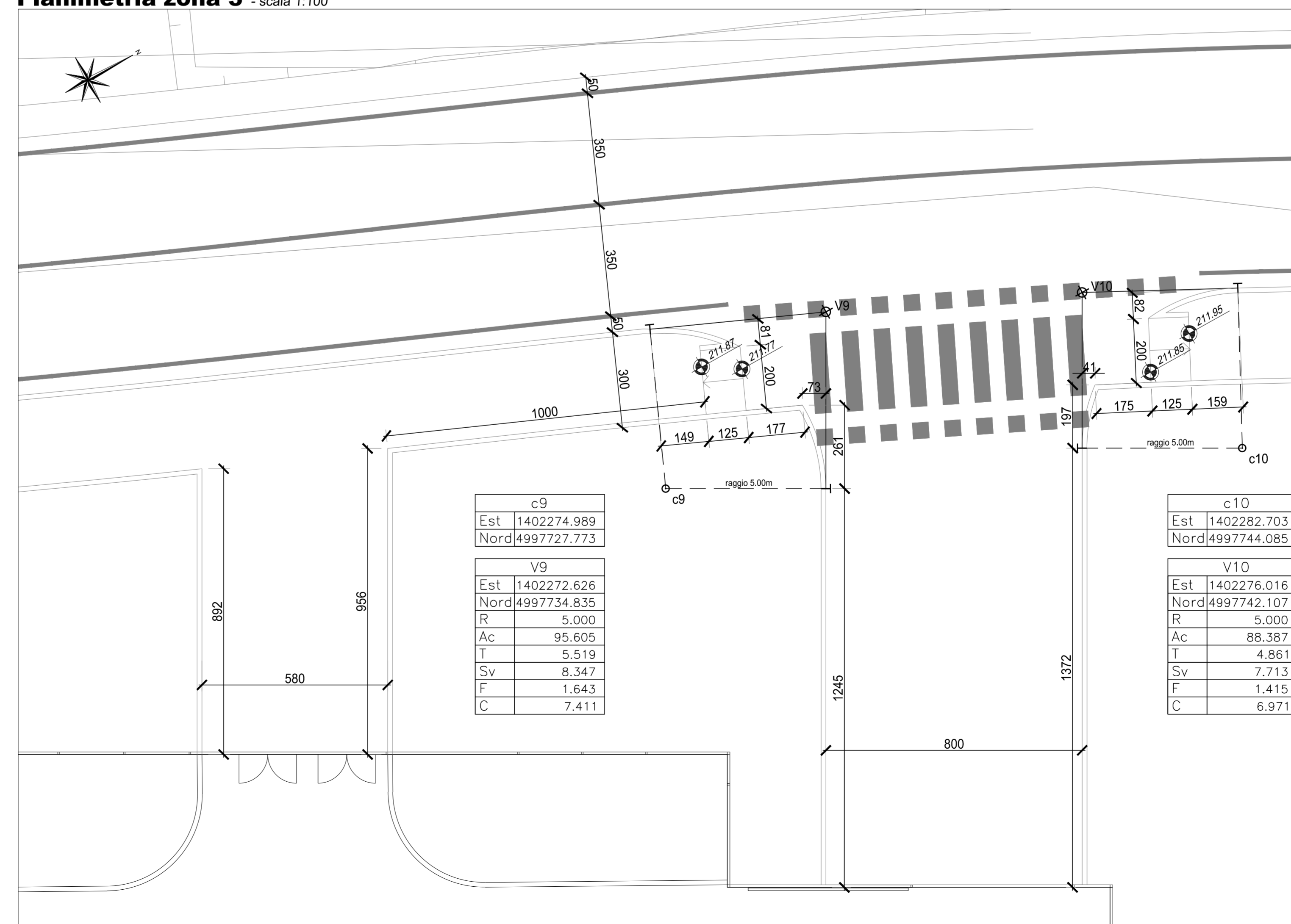
Planimetria zona 3 - scala 1:100
