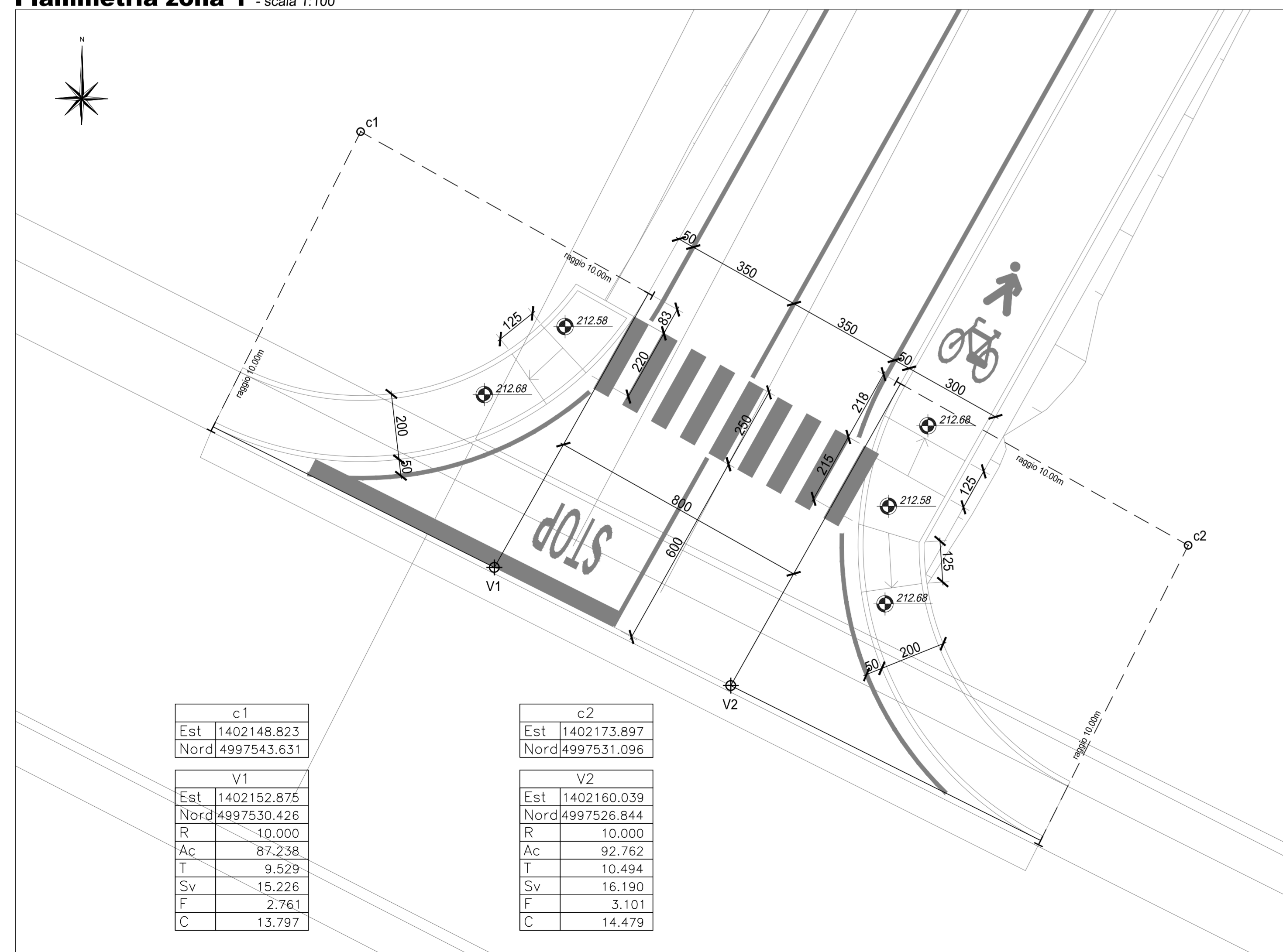
Planimetria zona 1 - scala 1:100
